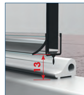
Art.-Nr. 8876KU0-12-2500 für 10 und 12 mm Glas
