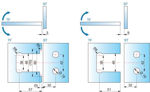
Glasbearbeitungen für die unterschiedlichen Spaltmaße
