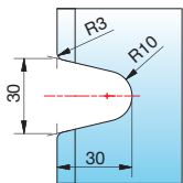
Randausschnitt R30
