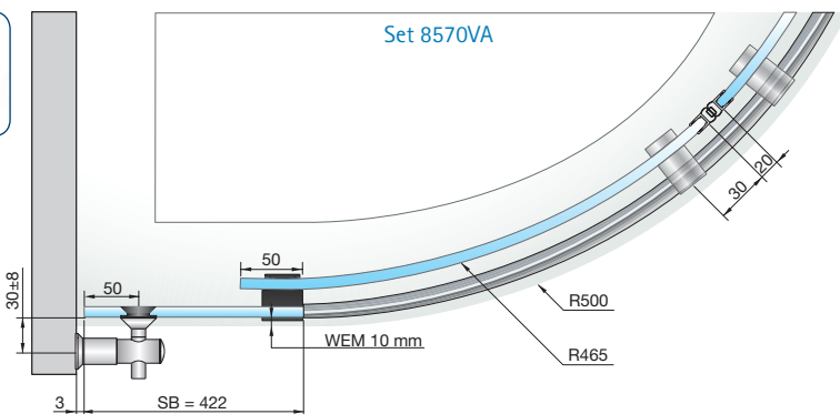
Set 8570VA: Einfachlaufrohr, Runddusche, Wandhalter flächenbündig, für Duschtasse 900 x 900 mm, R500
