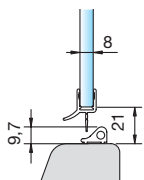
Art.-Nr. 8868KU0-8-R500 für 6 und 8 mm Glas in Verbindung mit gebogenen Schwallenschutzprofil für Wannenradius R500-550 Abwicklung = 1194 mm (Art.-Nr. 8881und 8882-R500)
