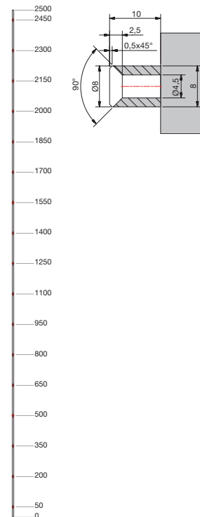
Trägerprofil für Dichtprofil
