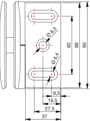
Befestigungslasche für 8418MS und 8430MS
