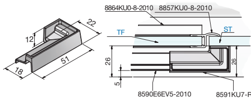
Art.-Nr. 8591KU7-R Abdeckkappe rechts
