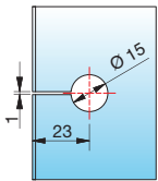
Bohrlochmaß bei 100°
