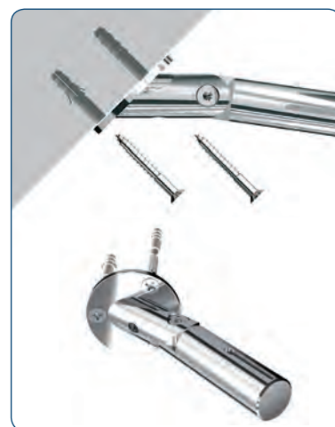
Wandanschluss 8576VAR mit Wandanschlussplatte 8545-1VA und Schraube S7991A2D8x16
