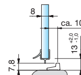
Art.-Nr. 8879KU0-8-2010 Für 8mm Glas in Verbindung mit dem Schwallenschutzprofil Art.: 8590E6EV5-2010 Achtung! Ist für den 90° Eckverbinder auszuschneiden, alle anderen Abdeck- kappen passen nicht!
