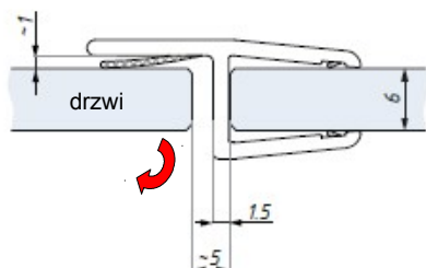
Uszczelka OWE6-8 montaż na szkło 6 mm Clip seal OWE6-8 for glass 6 mm
