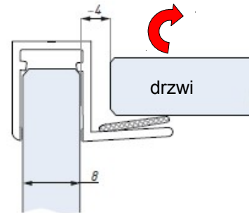
Uszczelka ASE6-8 montaż na szkle 8 mm Clip seal ASE6-8 for glass 8 mm
