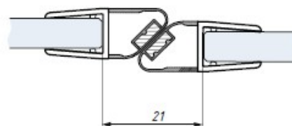
Uszczelka PMFE6-8 montaż na szkło 6 mm Clip seal PMFE6-8 for glass 6 mm
